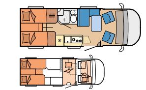
L: 6.759 mm · B: 2.230 mm H: 2.820 mm · G: 3.500 kg
